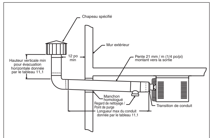
Figure 12,3 Évacuation horizontale de catégorie I - Té avec pente montante
